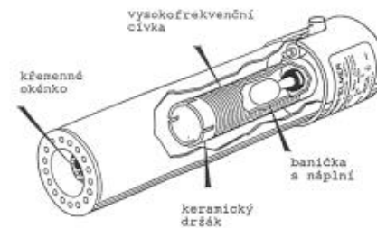
EDL výbojka f. Perkin Elmer (USA)
